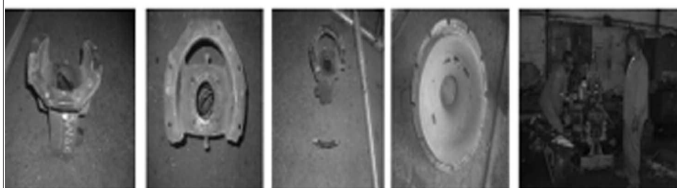
Corps de panier HS défectueuse et en train d'être usiné
